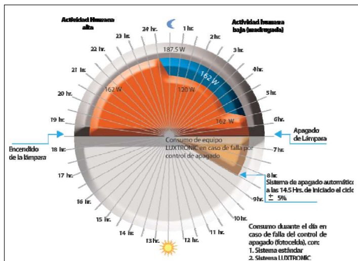
Gráfica comparativa de consumo durante 12 horas de trabajo para un sistema de 150W en un ciclo 651
